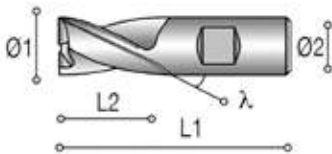
Spiebaanfrezen 2 lippen - SF2L
