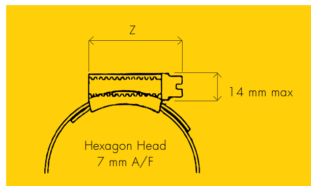
Afmetingen standaard slangklemmen
